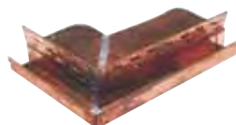
Kiesfang bei Balkonrinnen
