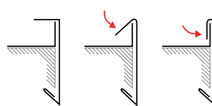
Stirnbrettverkleidung durch Rollenwechsel in 2 Arbeitsschritten (bei breiteren Einkantungen)
